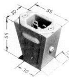
Тип КО-11A, C22, 16A, 250V, за нагреватели от \varnothing 40-99 мм 40-до \varnothing 99 мм
