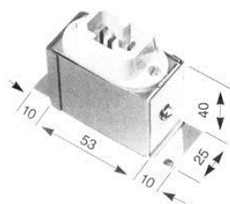
Тип КО-STE C16, 10A, 250V, за нагреватели по големи от \varnothing 75 мм
