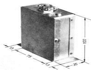
Тип КА-16: 40А, 2-полюса, за нагреватели \varnothing 100 мм или по-голям
