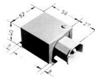
Тип КО-11B, C22, 16A, 250V, за нагреватели по-големи от \varnothing 75 мм 75мм
