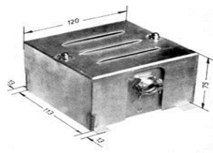
Тип КА-20 / 3: 3x40А, 3-полюса, за нагреватели \varnothing 150 мм или по-голям
