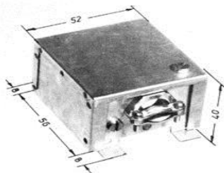
Тип КА-13: 16А, 2-полюса, за нагреватели \varnothing 75 мм или по-голям
