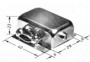
Тип КА-22: Твърда кабелна връзка- само за плоски нагреватели или повърхности.
