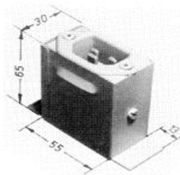
Тип КО-11, C22, 16A, 250V, за нагреватели по- големи от \varnothing 100 мм
