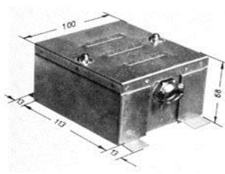
Тип КА-19: 40А, 2-полюса, за нагреватели \varnothing 150 мм или по-голям
