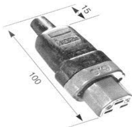
C21, 16A, 250V, силиконов щепсел
