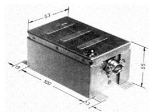
Тип КА-18: 30А, 2-полюса, за нагреватели \varnothing 150 мм или по-голям
